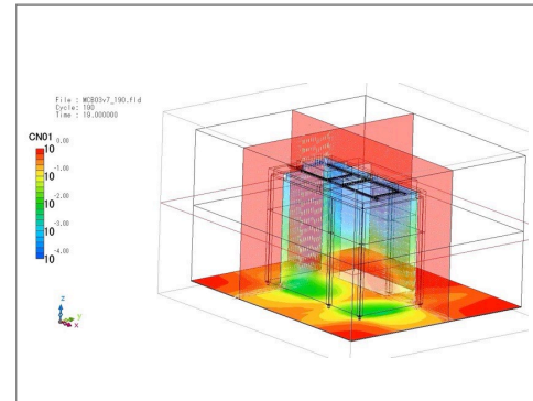
気流解析
